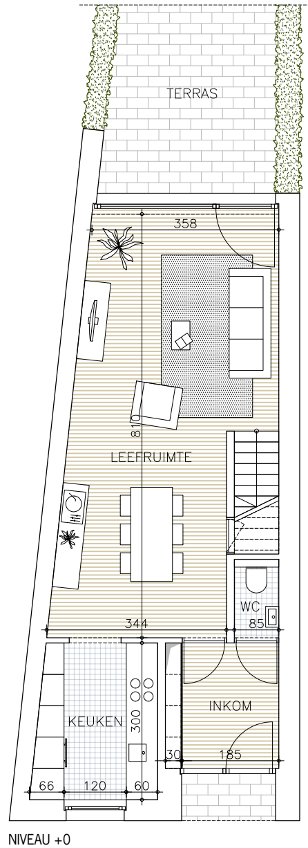
NIVEAU +0
