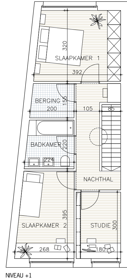
NIVEAU +1
