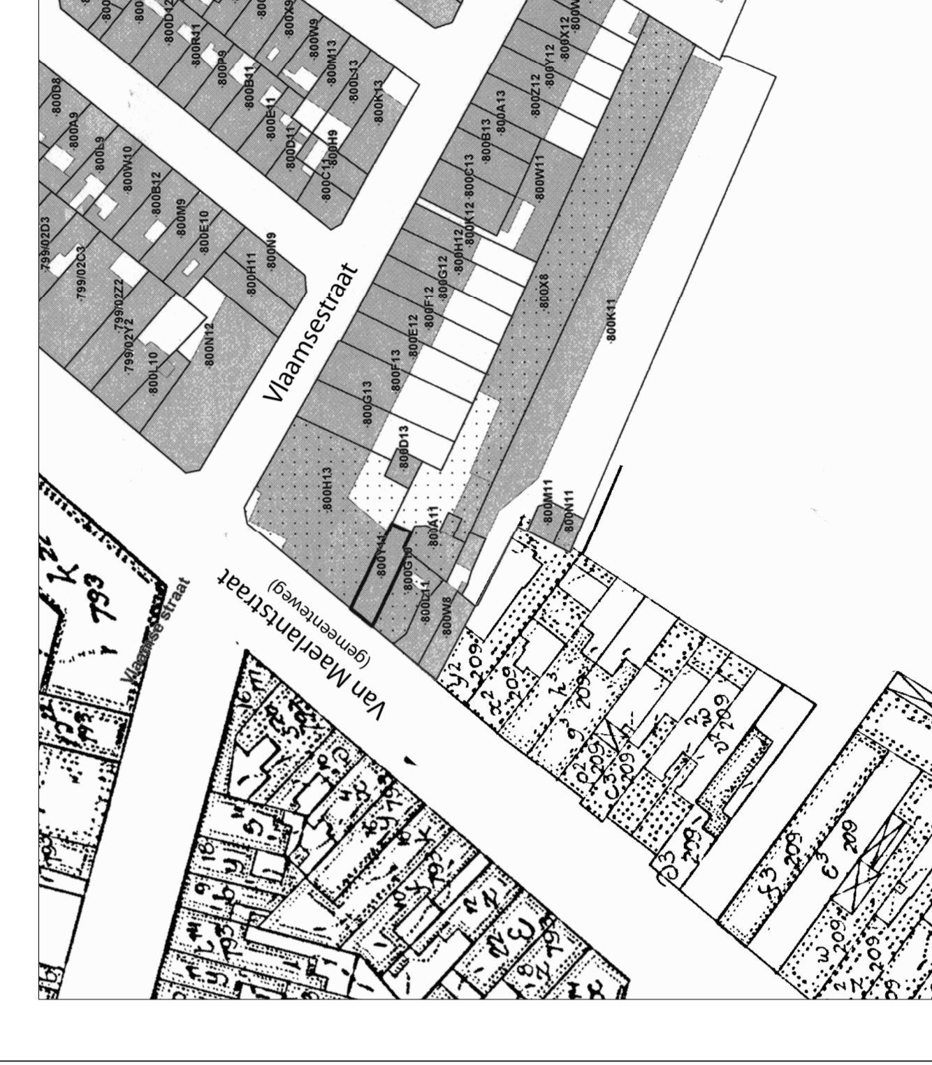
OMGEVINGSPLAN schaal 1/750
