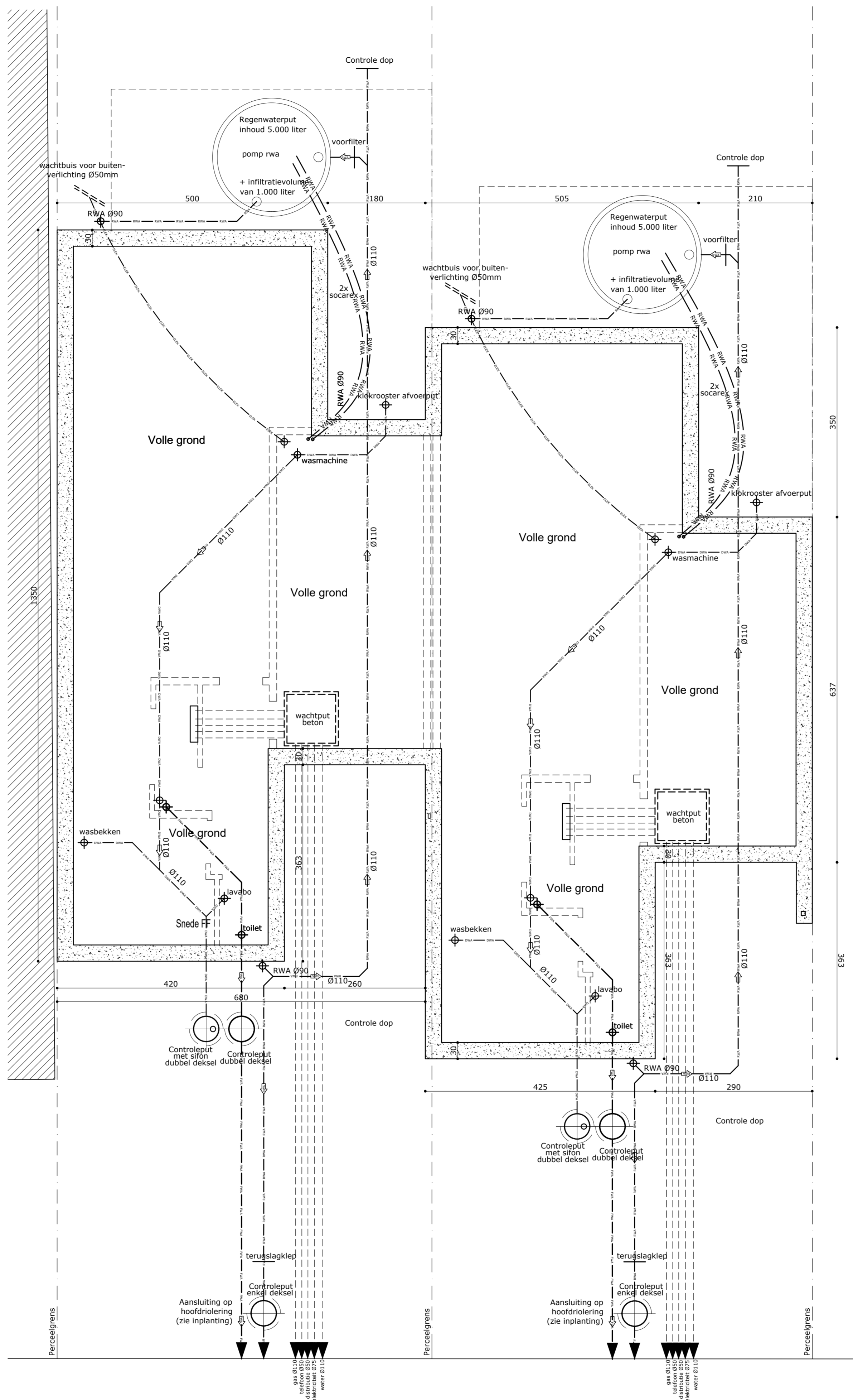
rioleringsplan blok A 1/50
