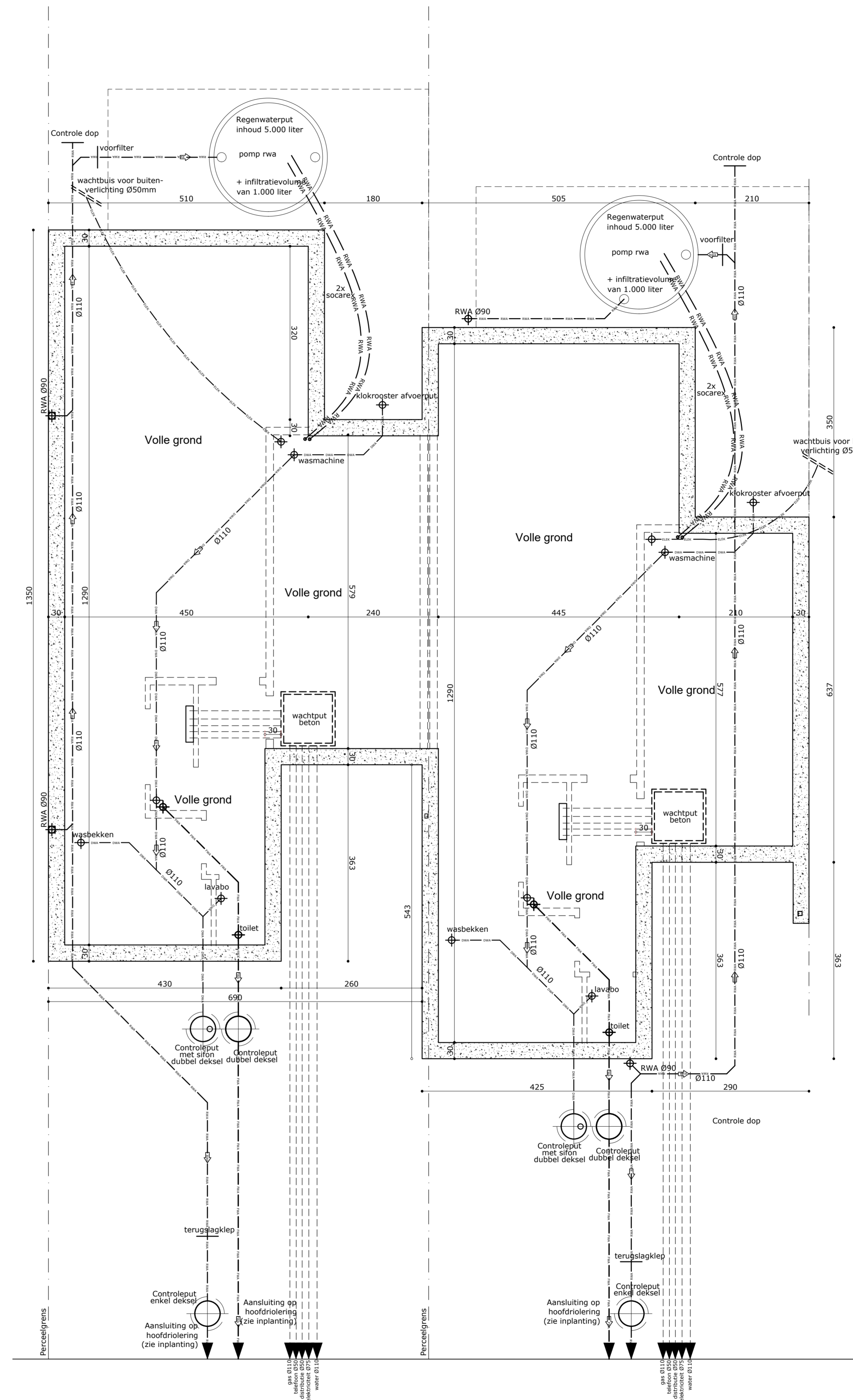
rioleringsplan blok B 1/50
