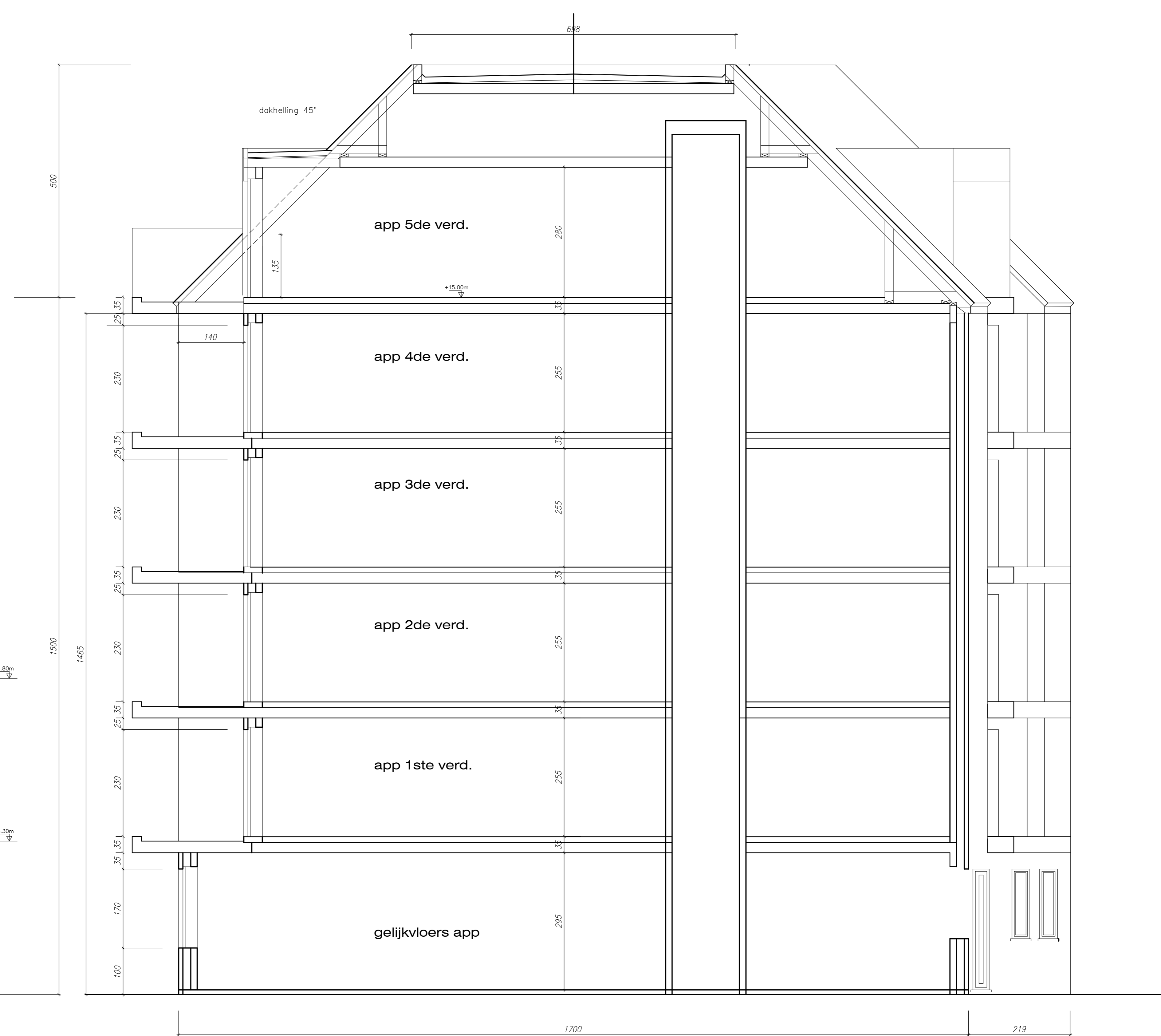
doorsnede
