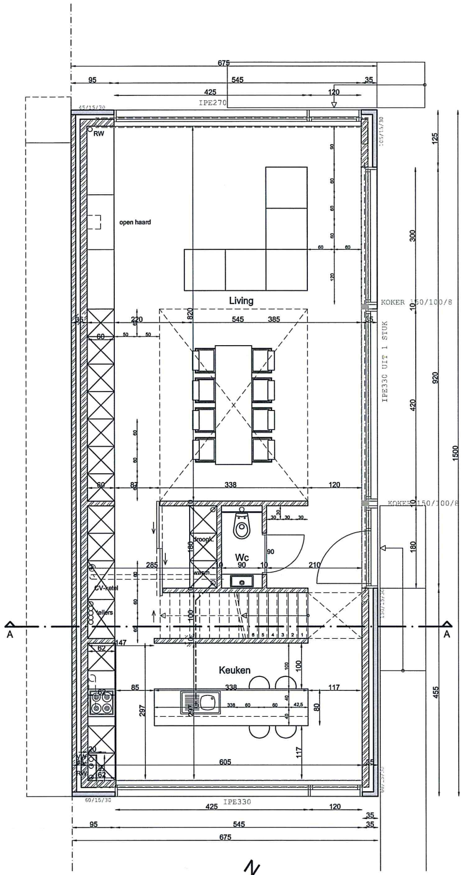
Grondplan
